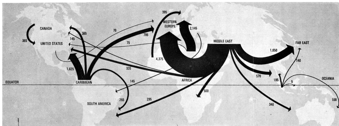
Planche 34 Les exportations des pétroles du Moyen-Orient, d'Amérique et d'Asie du Sud-Est, en milliers de barils par jour, en 1969. Par la suite de leur dilapidation, aggravée en 1970-1971, il est probable que le prix du pétrole soit doublé ou triplé avant 1976. Le calcul des probabilités fixe également vers 1982 l'arrêt presque total des exportations des carburants du Moyen-Orient vers l'Occident, où les moteurs à combustion cesseront d'être alimentés en pétrole. Avions et autos seront immobilisés. Au dessus du 45° degré de latitude Nord (Limoges-Milan) les conditions du froid, intensifié par la pollution atmosphérique, rendront inhabitables les grands ensembles, palaces de verre, les stations de sport d'hiver, etc., tributaires du chauffage au mazout. Les populations nordiques tendront à émigrer vers le Sud : la Méditerranée, l'Afrique... plus tempérées.
